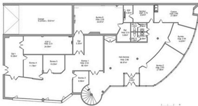
Niveau 0
